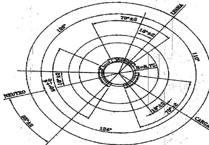
VISTA INFERIOR
