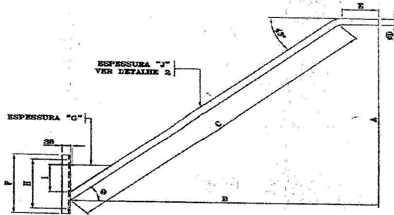
VISTA LATERAL
