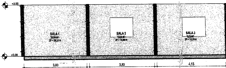
3 C - C 1:75
