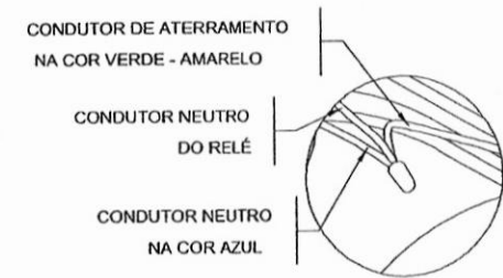
DETALHE 4 CONEXÃO DOS CONDUTORES DE ATERRAMENTO É NEUTRO
